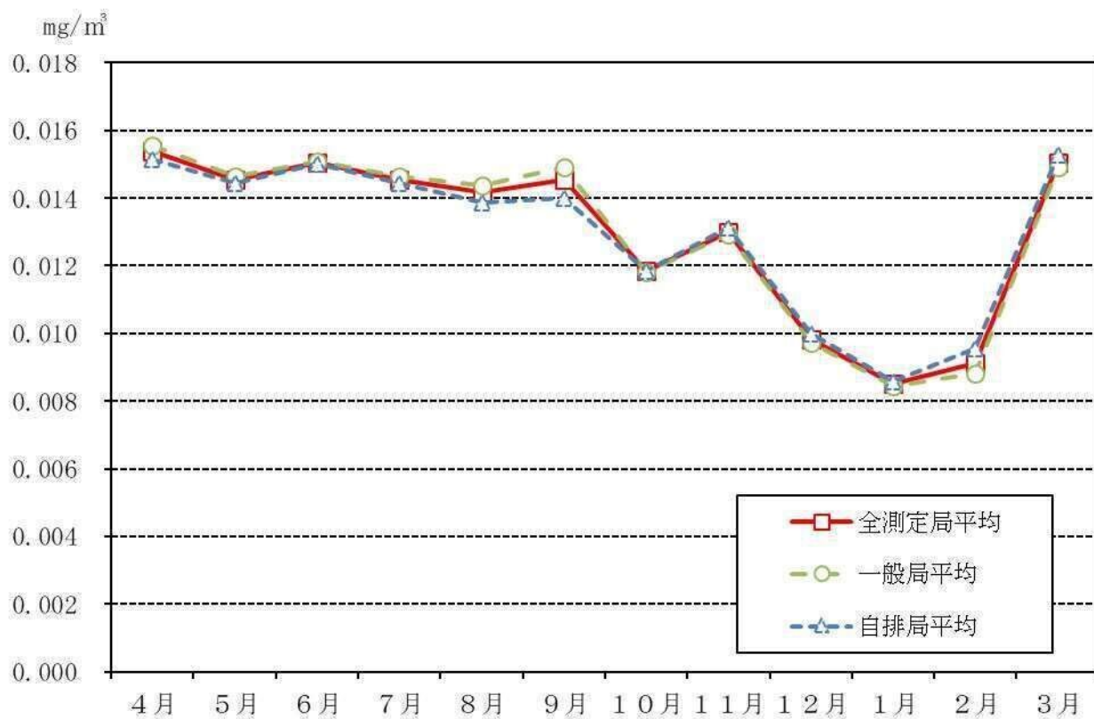
図 3-4-2 浮遊粒子状物質月平均値の市内平均経月変化（令和 3 年度）
