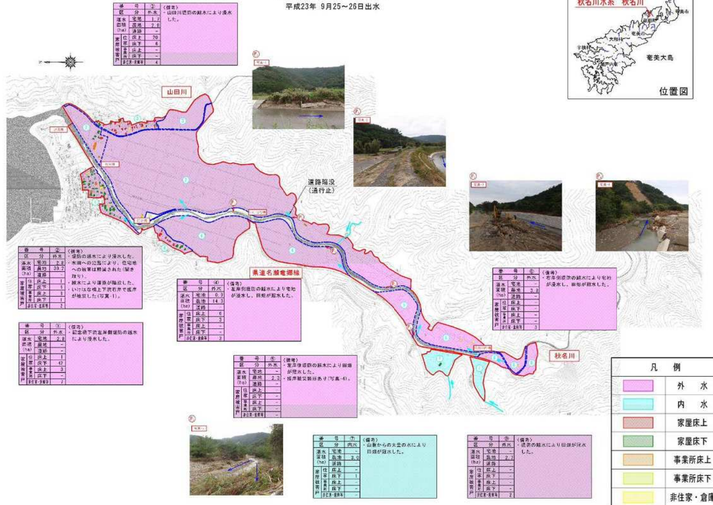
秋名川 浸水説明図
