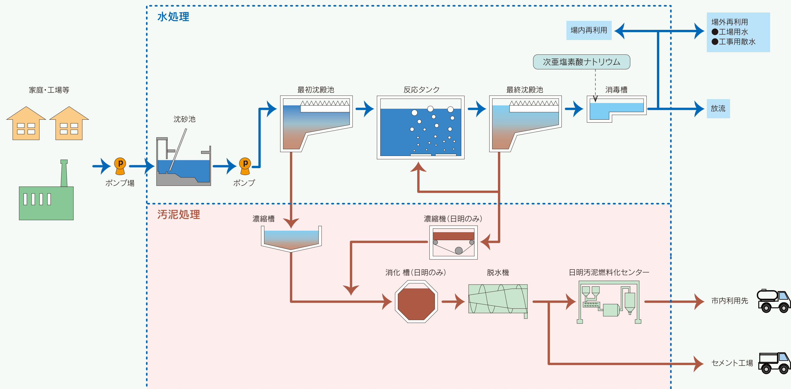
沈砂池
