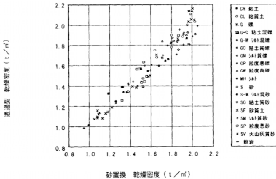
図一6 砂置換と透過型の相関（乾燥密度・土質別データ）
