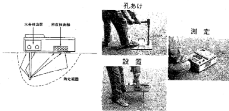
② 透過型
