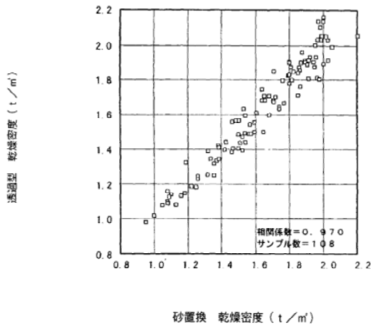
図一5 砂置換と透過型の相関（乾燥密度・全データ）
