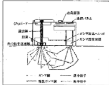
① 散乱型
